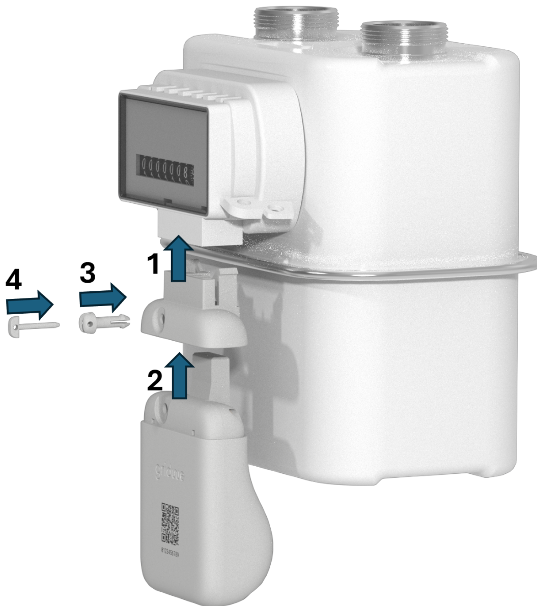
Рисунок 4 – Послідовність монтажу модемів
