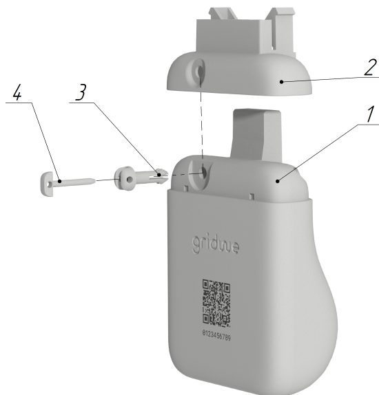
Рисунок 2 - Конструкція модему
