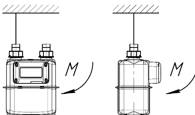
Рис. 6. Згинальний момент, що діє на лічильник при установці
