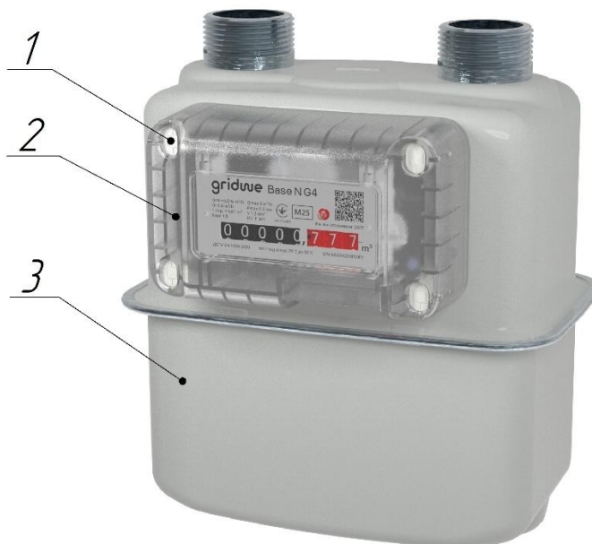
Рисунок 2 – Конструкція лічильника
